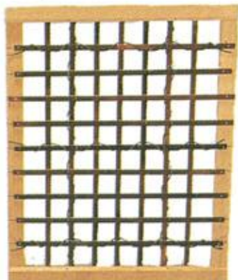
煤竹合せ下地窓
